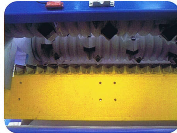
CUCHILLAS MÓVILES MONTADAS SOBRE HÉLICE
